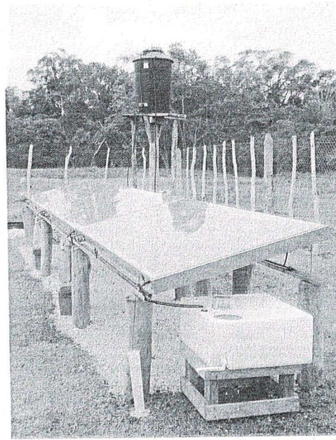
Diese solarbetriebene Wassergewinnungsanlage an der Mündung des Rio Maxima auf Kuba liefert Trinkwasser für 150 Menschen.
